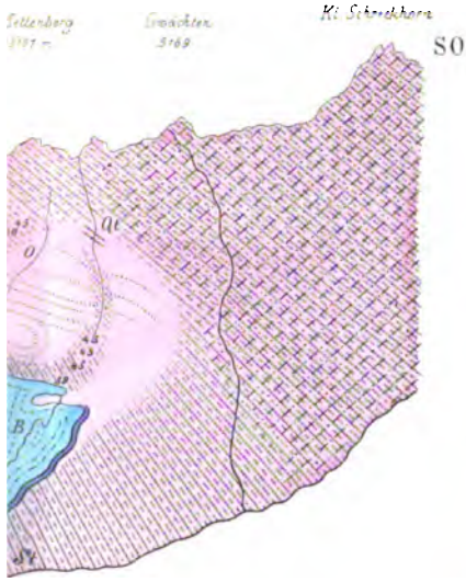
Teil am Meltenberg (Südwestseite) Bartholinus, J. - Jagdgräfli 2473 m. kont. Sch. - Schafalstein, St. - Steregg. von der Gneiss bedeuten den Fallwinkel
